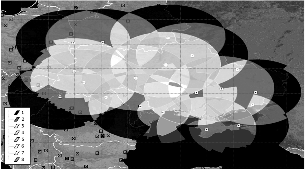
Рис.1. Результати оцінювання доступності далекомірних радіомаяків
