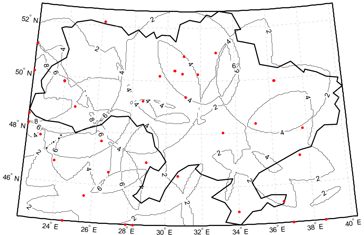
Рис. 3. Доступність DME/DME навігації для повітряного простору України
