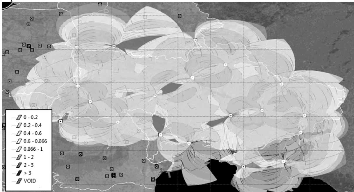
Рис.2. Результати оцінювання точності позиціонування за радіомаяками DME
